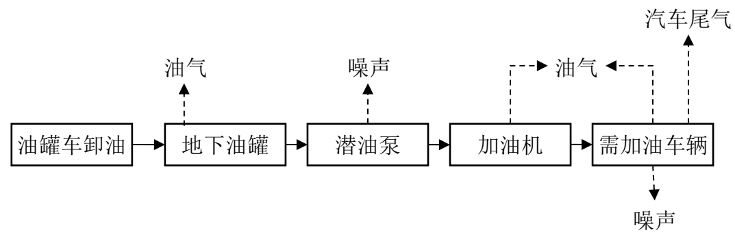
图 2 柴油加油工艺流程及产污环节示意图
